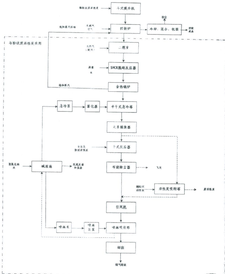
颗粒状废活性炭再生工艺流程
